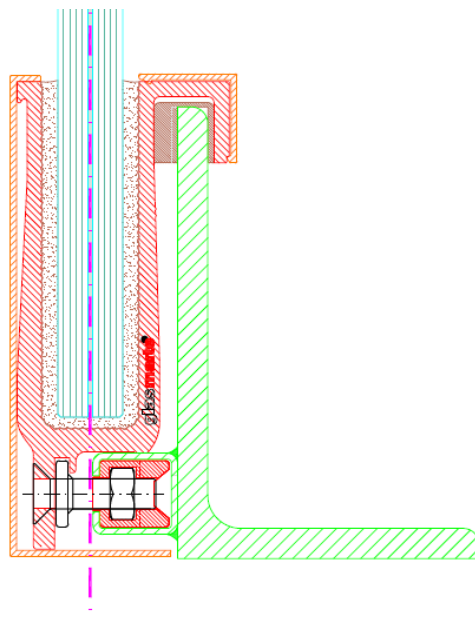
Abbildung 1: Vertikalschnitt der Konstruktion
